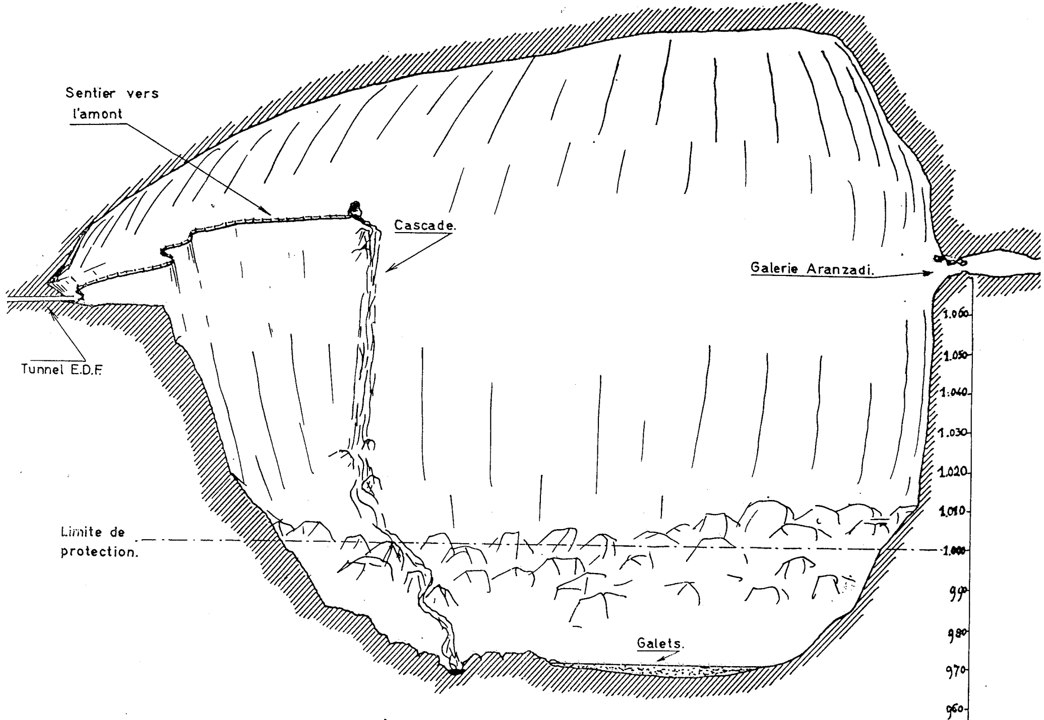
Salle de La Verna (coupe)
